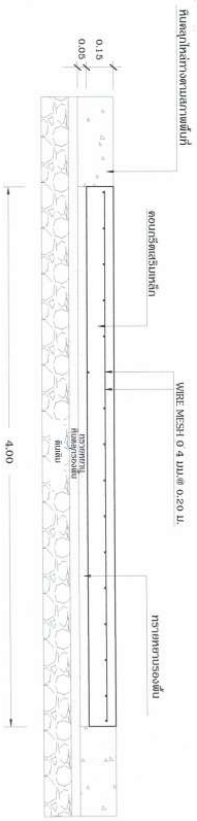
รูปตัด 1-1
